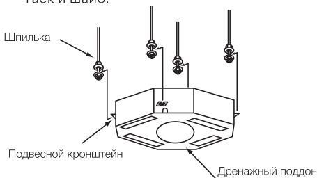
Установка внутреннего блока.
