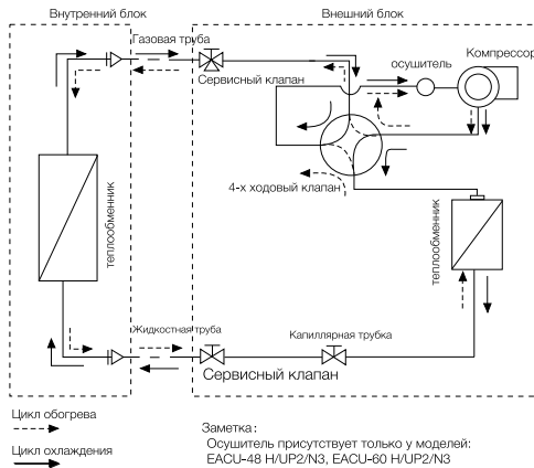
Внешний блок
