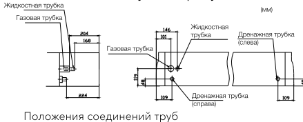
Положения соединений труб
