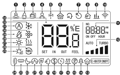
Обозначения на ЖК-дисплее:
