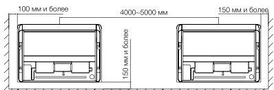
Установка под потолком
