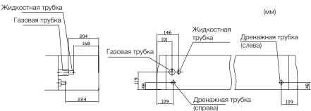
Положения соединений труб
