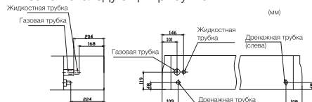
Положения соединений труб
